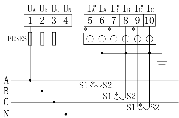
三相四线3CT
