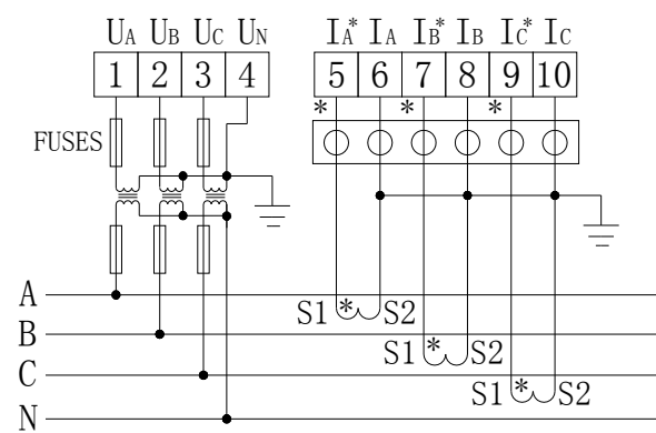
三相四线3PT、3CT
