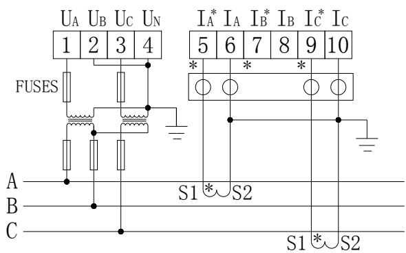
三相三线2PT、2CT
