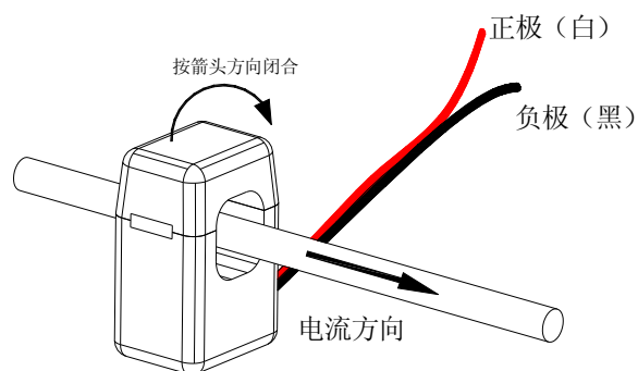
开口式互感器安装方式
