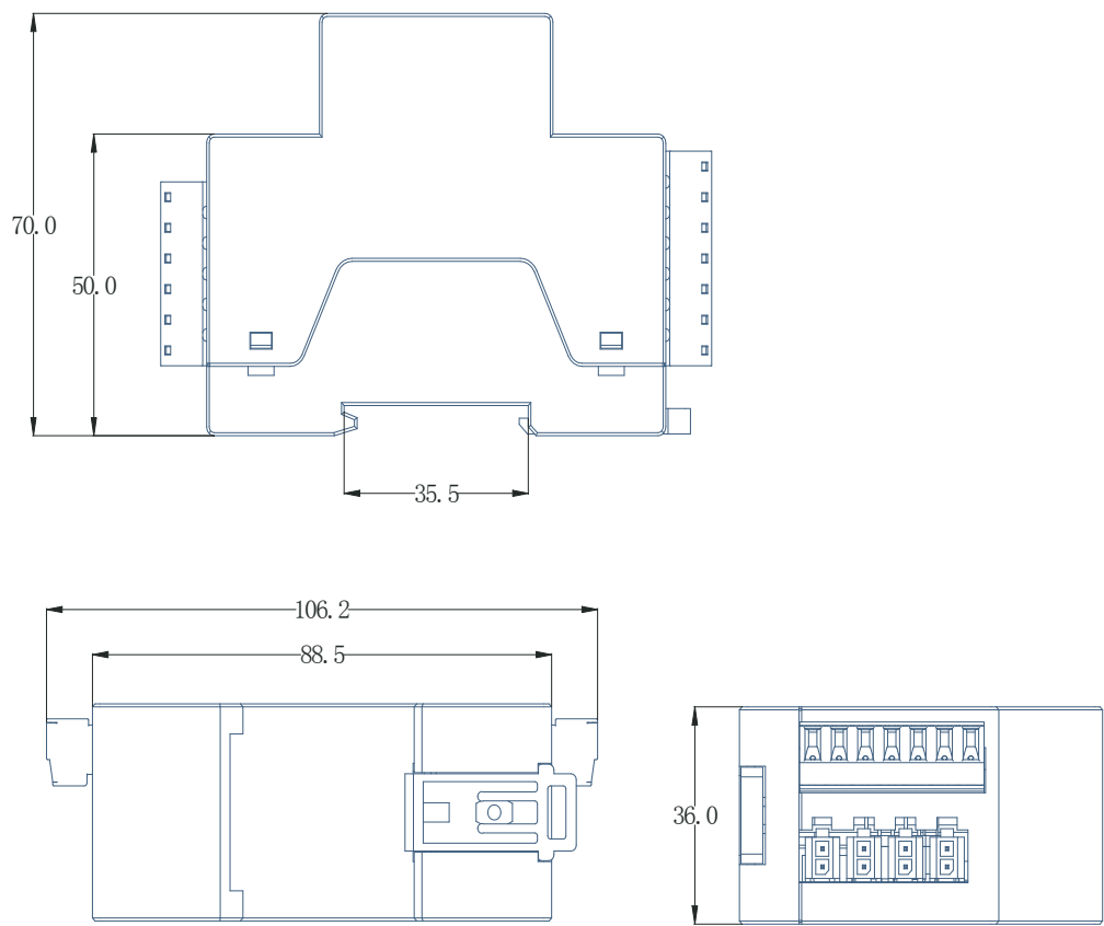
(1) ADW100 尺寸图
