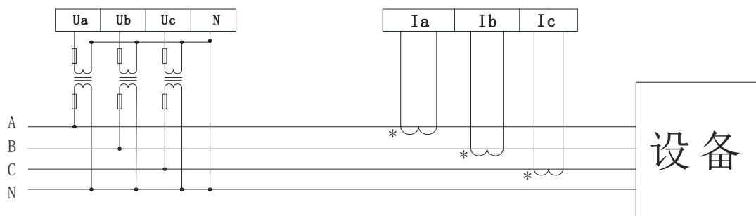
三相四线(电压经互感器接入)
