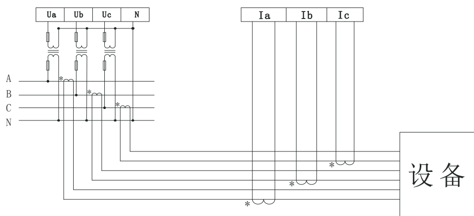
三相四线 (电压经互感器接入)
