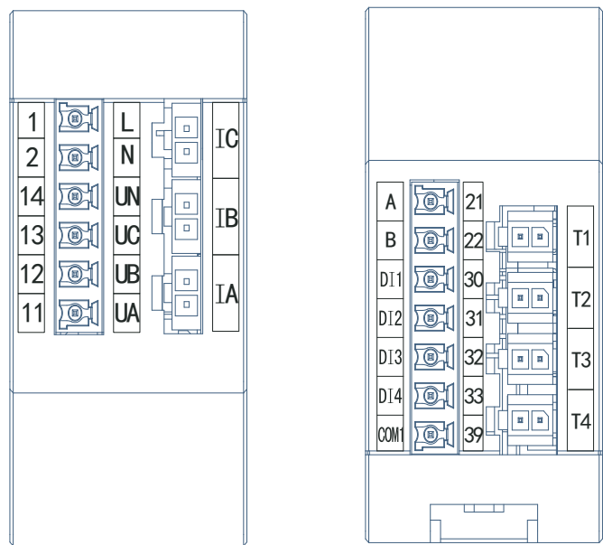
图 5 主体接线端子
