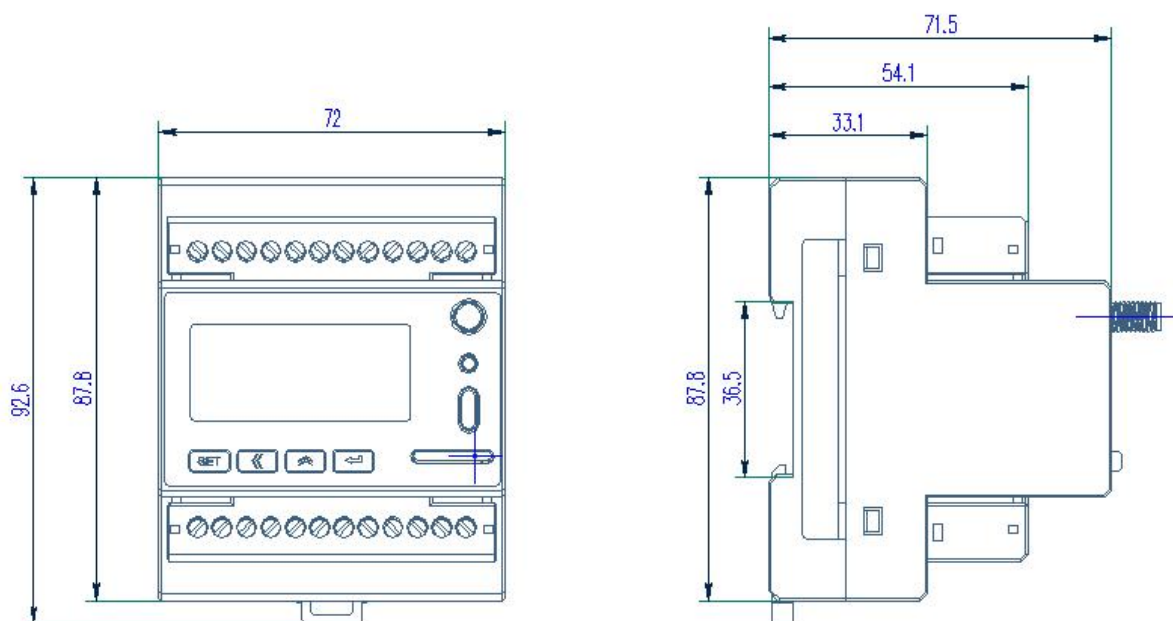
图 2 ADW300 尺寸图
