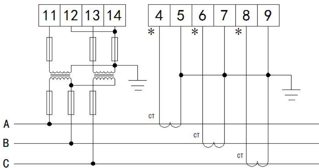
三相三线
