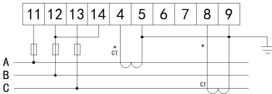
三相三线
