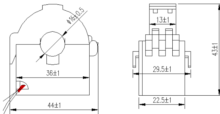
外置互感器尺寸（单位 mm）
