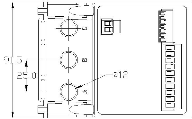
俯视图
