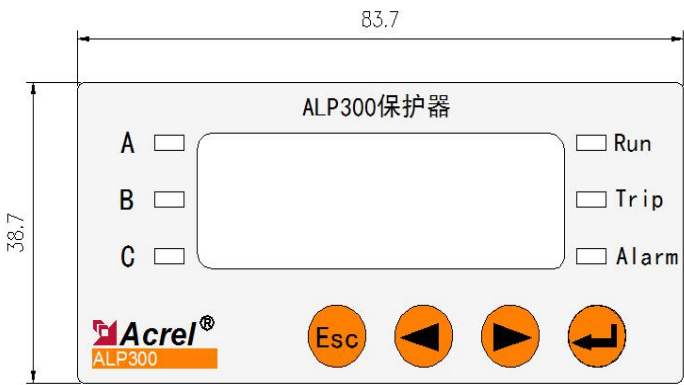
主视图
