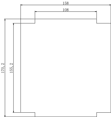
开孔尺寸
