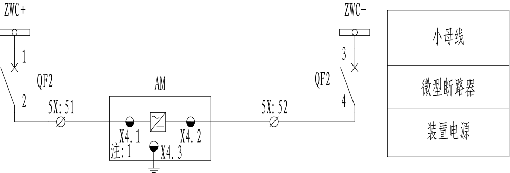
图 1.20 AM4-I（默认模式） 二次原理图（一）
