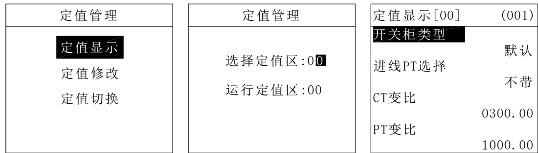
图 3.9 定值菜单
