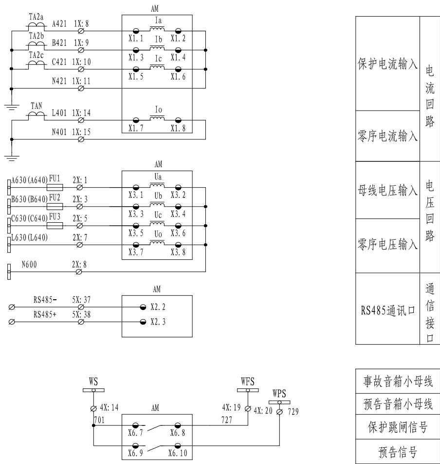
图 1.22 AM4-I（默认模式）二次原理图（三）
