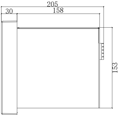
侧视图
