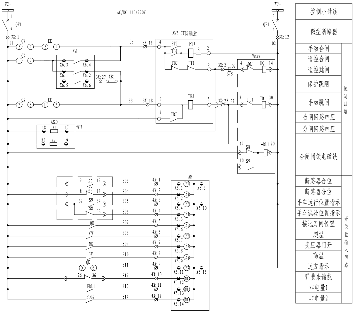
图 1.21 AM4-I（默认模式）二次原理图（二）
