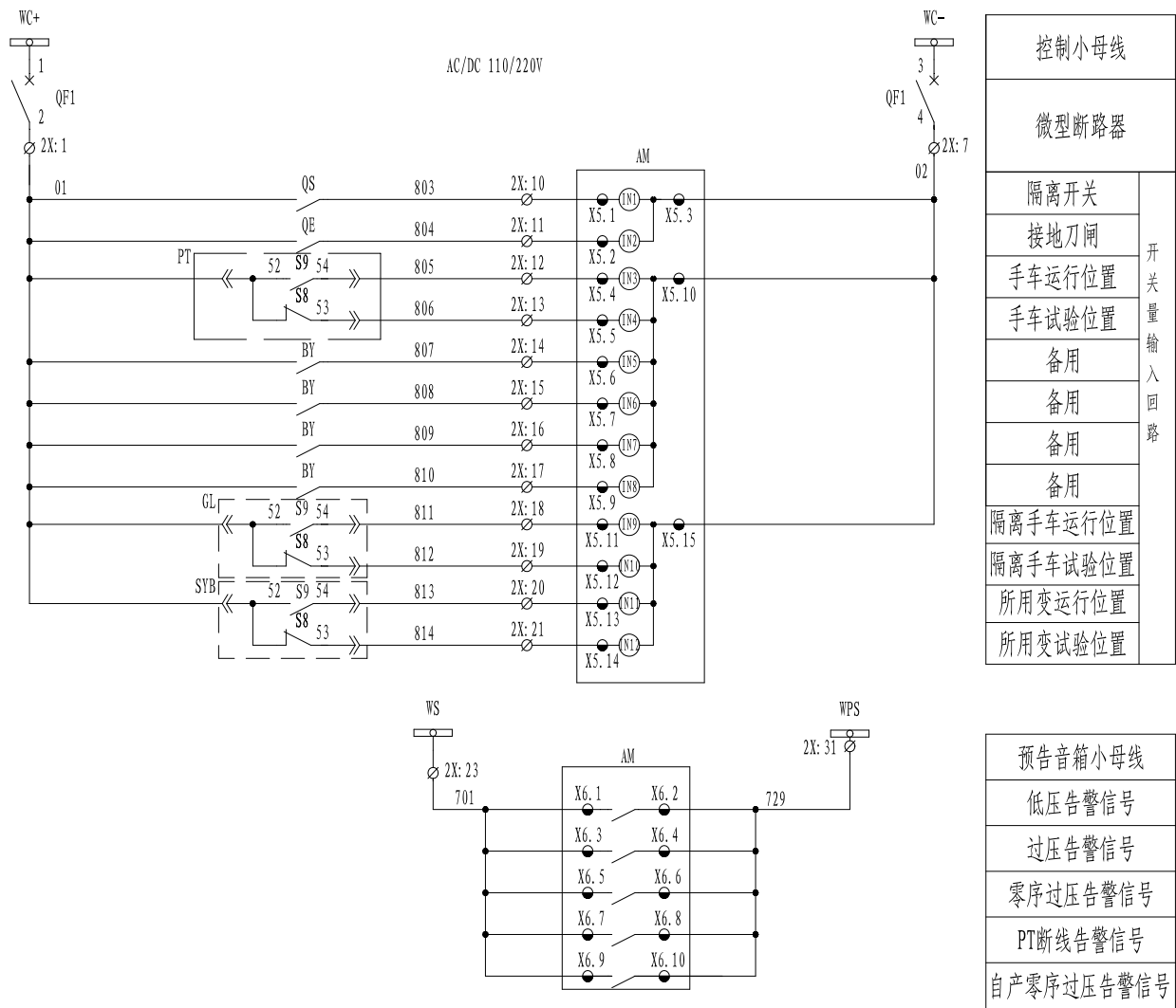
图 2.10 AM4-U1 二次原理图（三）
