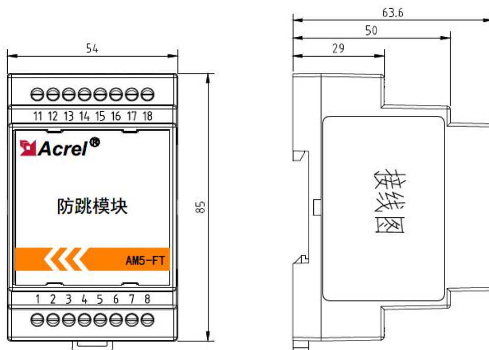
图 1.3 AM5-FT 尺寸图
