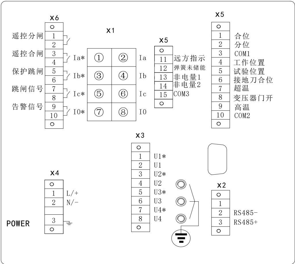
图 1.18 AM4-I（默认模式） 电气接线图
