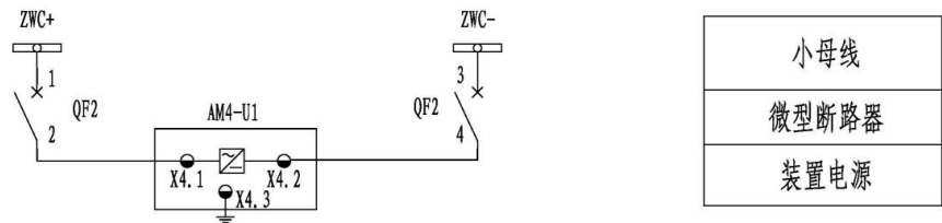
图 2.8 AM4-U1 二次原理图（一）
