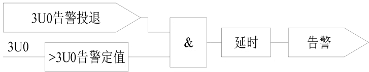
图 2.5 零序过压告警逻辑
