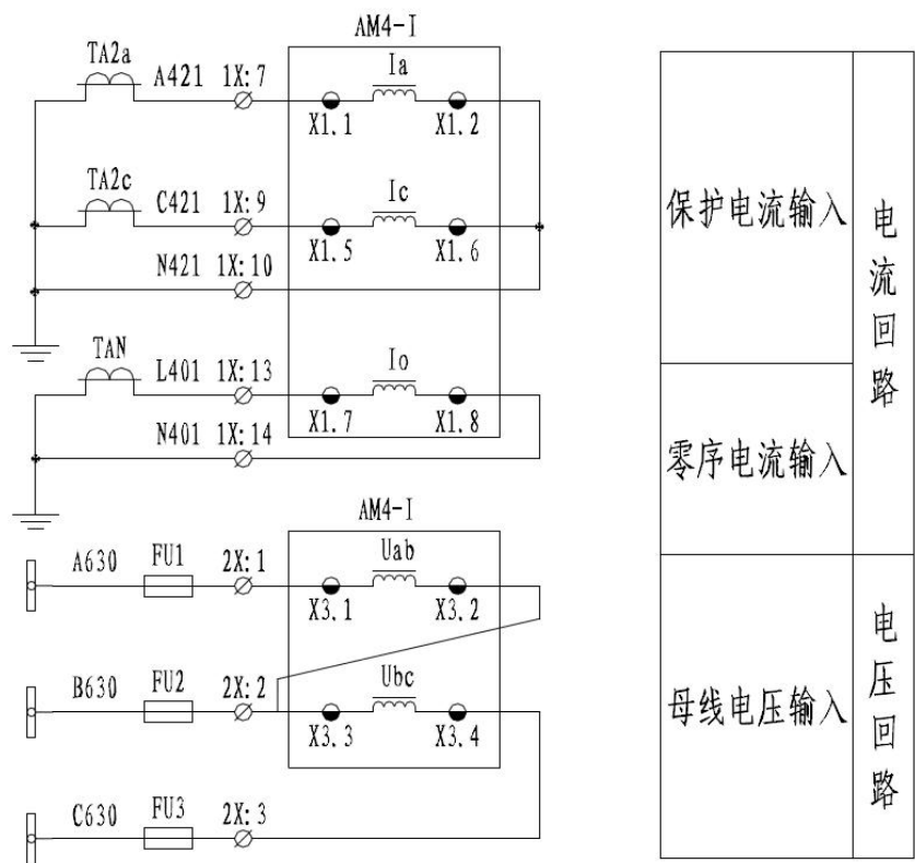
图 1.19 2PT 2CT 接线方法
