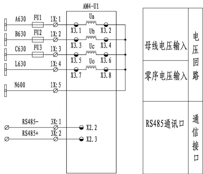
图 2.9 AM4-U1 二次原理图（二）
