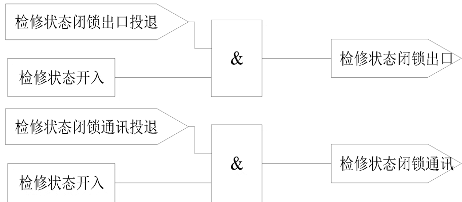
图 1.17 检修状态闭锁逻辑
