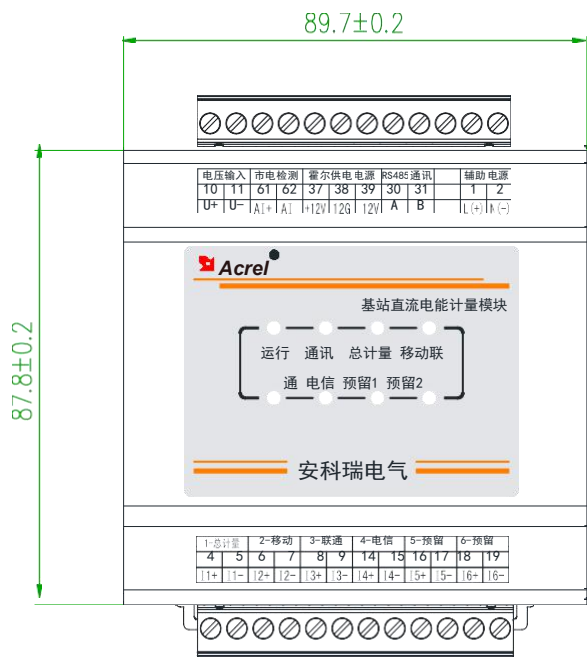
模块主视图
