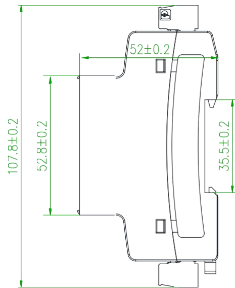
模块左视图
