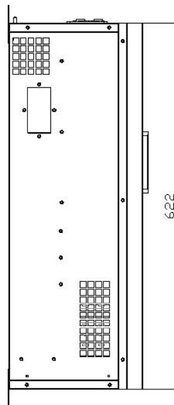
图 2-6 ANSVG-50kvar、ANSVG-75kvar 壁挂模块机箱侧视图
