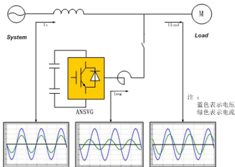
图2-18 ANSVG 原理图
