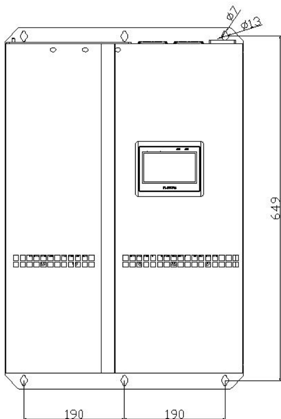
图 2-5 ANSVG-50kvar、ANSVG-75kvar 壁挂模块机箱主视图
