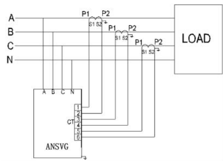
图 4-1 电流互感器安装位置及单 ANSVG 电流互感器接线示意图
