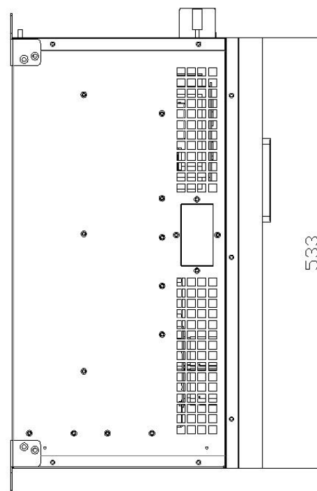
图 2-12 ANSVG-100kvar 壁挂模块机箱侧视图
