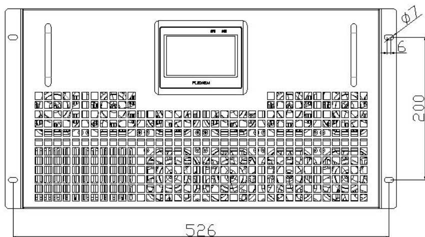
图 2-8 ANSVG-100kvar 模块机箱主视图
