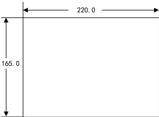
图 1.5 ASD200、ASD300、ASD310、ASD320 开孔尺寸
