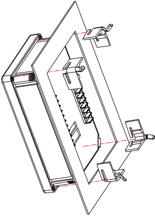
图 1.2 ASD100/ASD100G 安装方法
