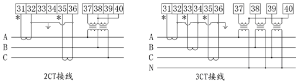
图 2.3 接线方式
