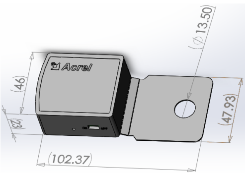
图 1.8 螺栓式无线温度传感器 ATE100
