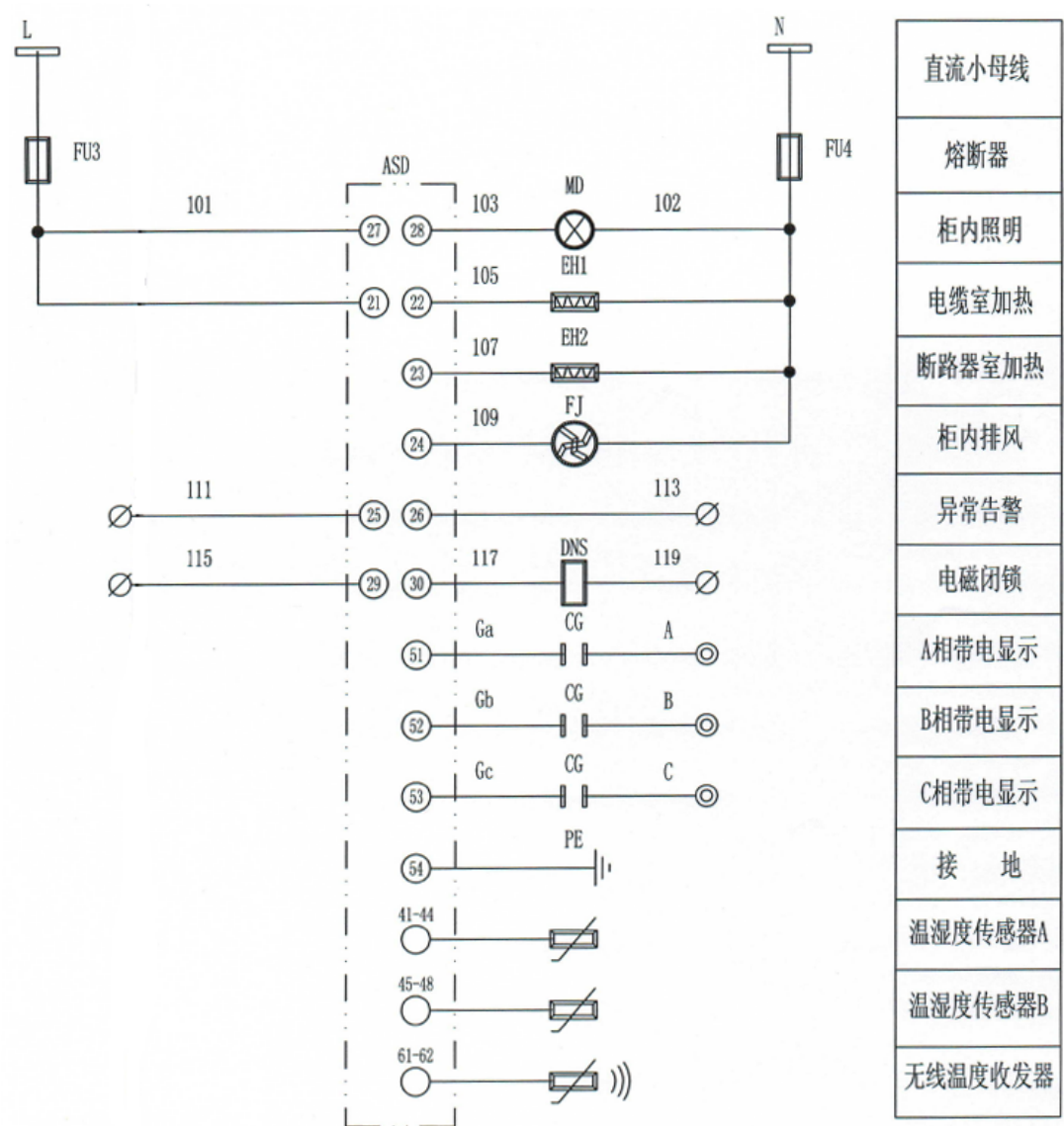
图 1.16 ASD 开关量输出、高压带电显示回路及传感器典型接线图
