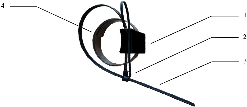
图 1.10 ATE300 结构说明
