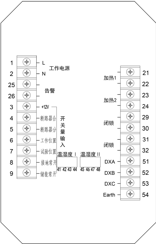
图 1.11 ASD100G 背面端子图
