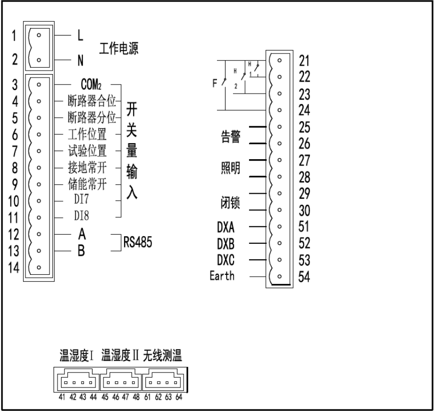
图 1.13 ASD320 背面端子图
