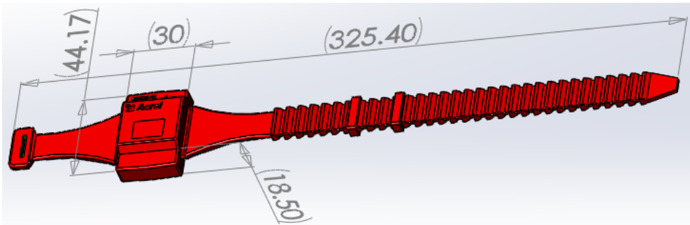
图 1.7 表带式无线温度传感器 ATE200
