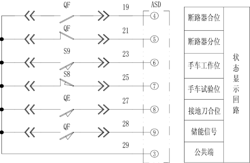
图 1.15 ASD 开关量输入回路典型接线图
