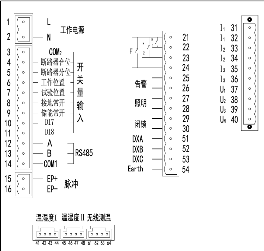
图 1.12 ASD300 背面端子图
