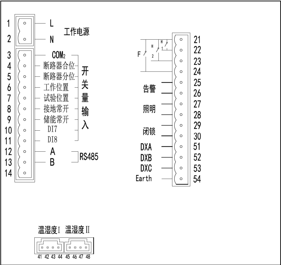
图 1.14 ASD200/310 背面端子图
