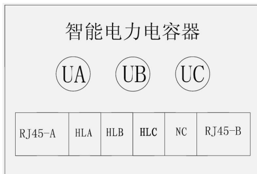
分补接线端子图
