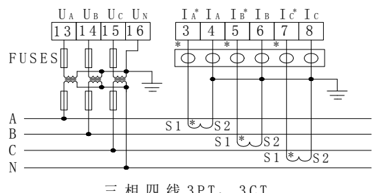
三 相 四 线 3PT、3CT
