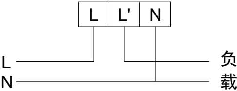
DDSF1352 接线图
