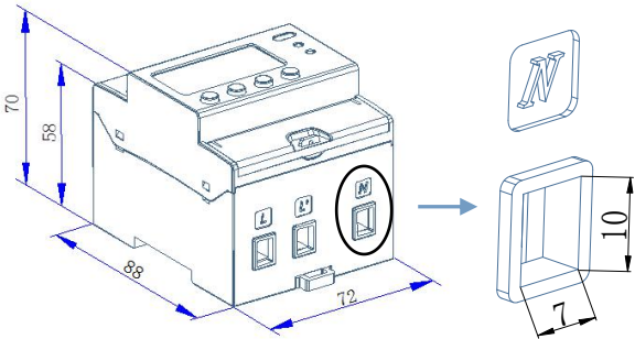
直接接入接线图
